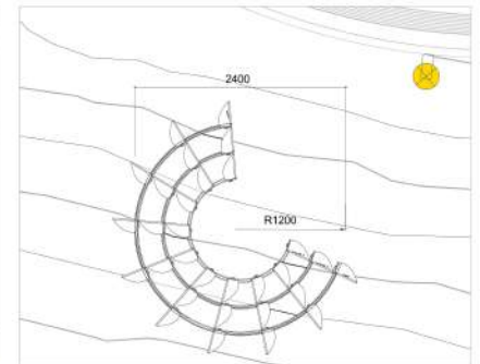
2 Planas A 1 : 50
