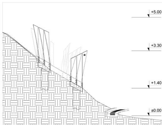
4 Pjūvis A 1 : 50
